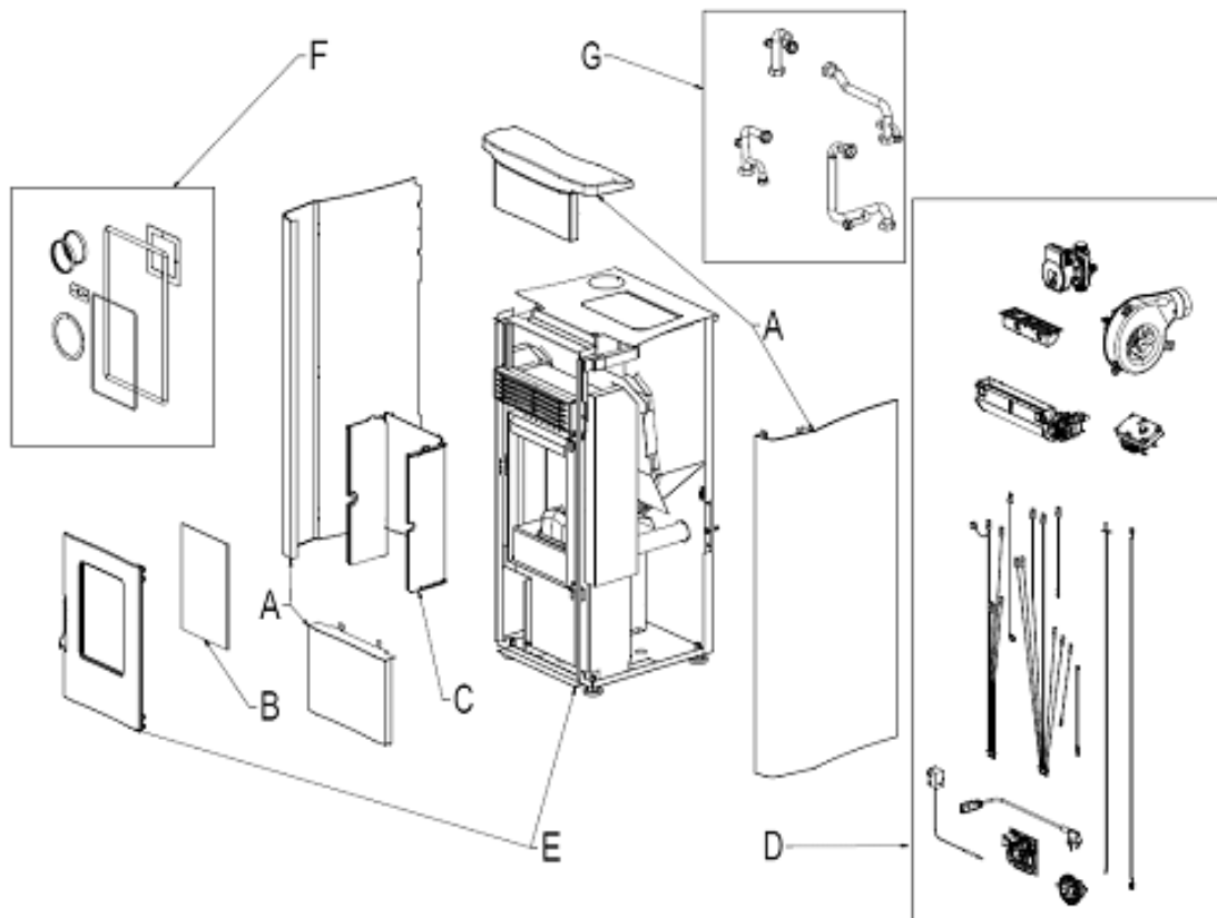
Fig. 1 - Geëxplodeerde tekening
